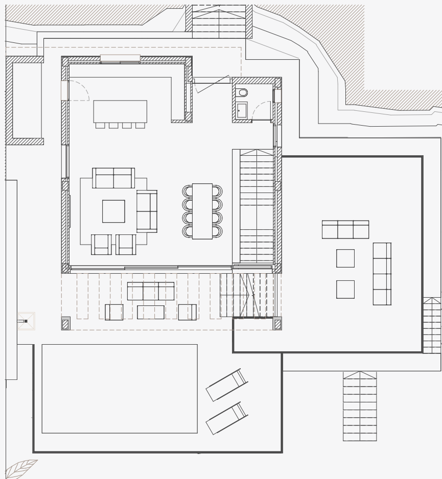
PRIMERA PLANTA
